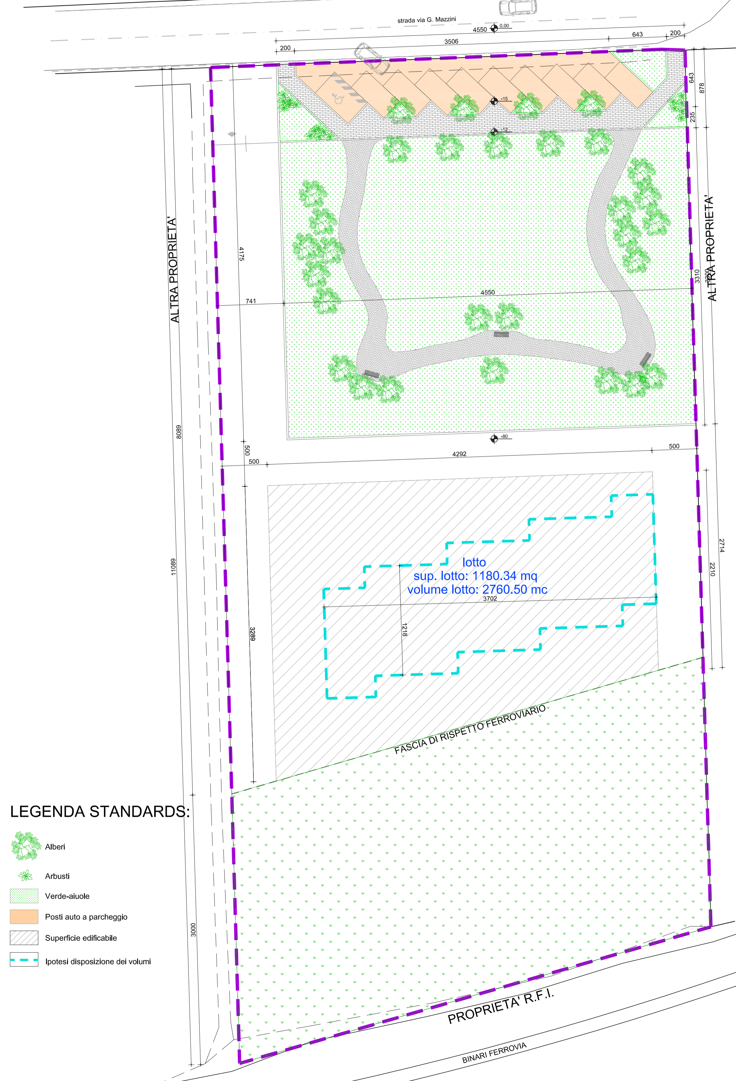
PLANIMETRIA QUOTATA delle SUPERFICI EDIFICABILI scala 1:250
